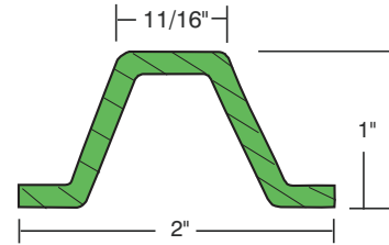
Rhino 112 (1.12 lbs. per lineal foot)
