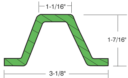
Rhino 200 (2.0 lbs. per lineal foot)
